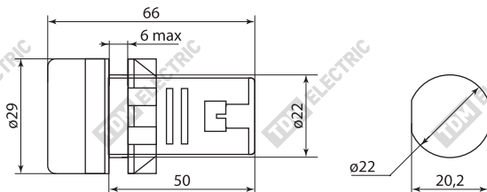
Рисунок 1. Габаритные размеры сигнализаторов, мм
